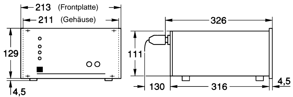
Abb. 2 Maßzeichnung, Maße in mm
